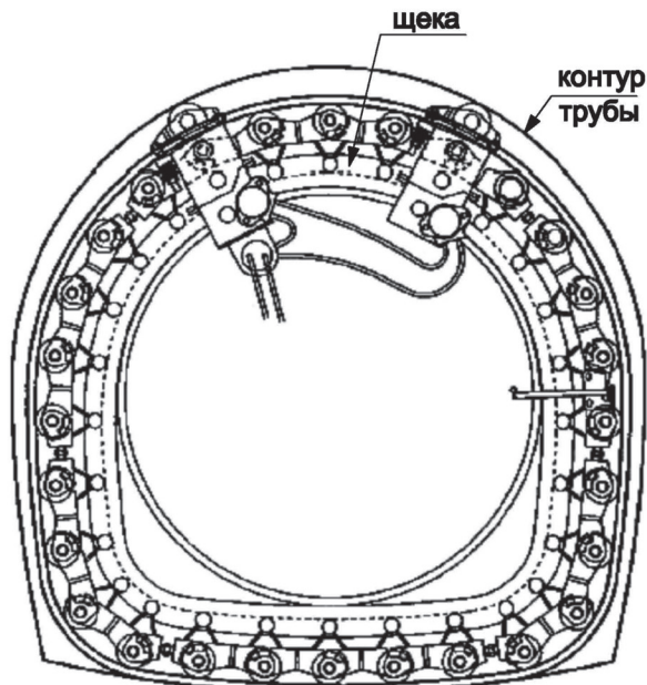
Рисунок 12 – Навивочная машина в собранном виде
